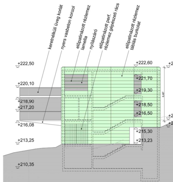
nyugati homlokzat
