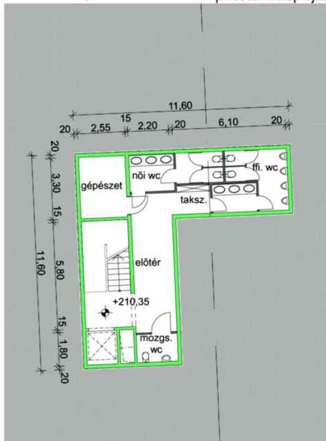
pincésint alaprajza
