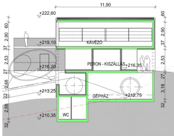
A-A metszet
