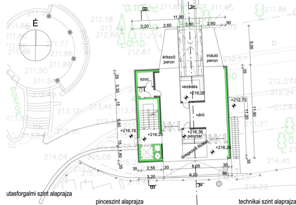
pincésint alaprajza
