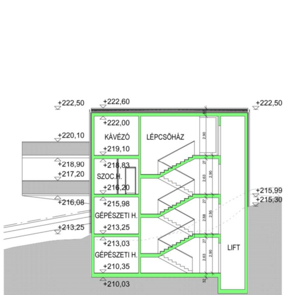
B-B metszet
