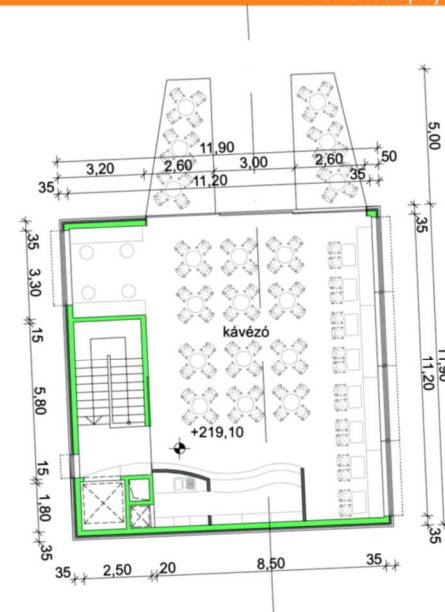
emelet alaprajza
