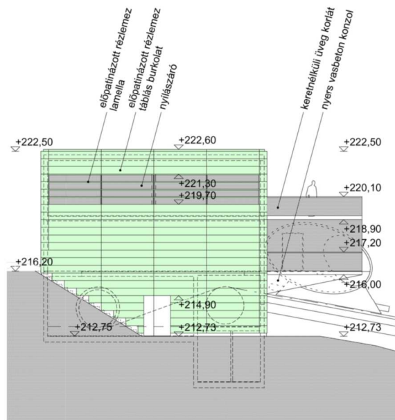
keleti homlokzat
