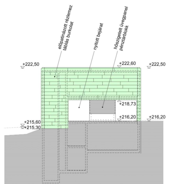
déli homlokzat
