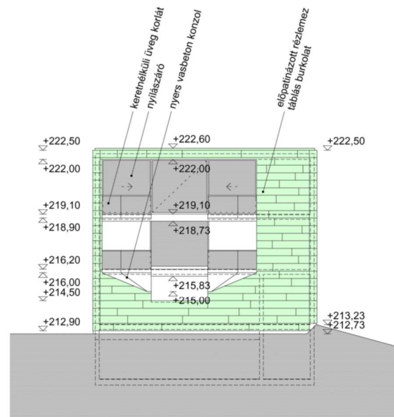
északi homlokzat
